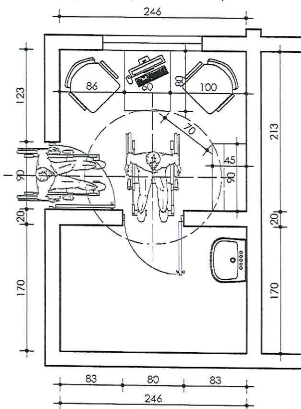
Plano con circunferencia de referencia para el acceso de silla de ruedas
